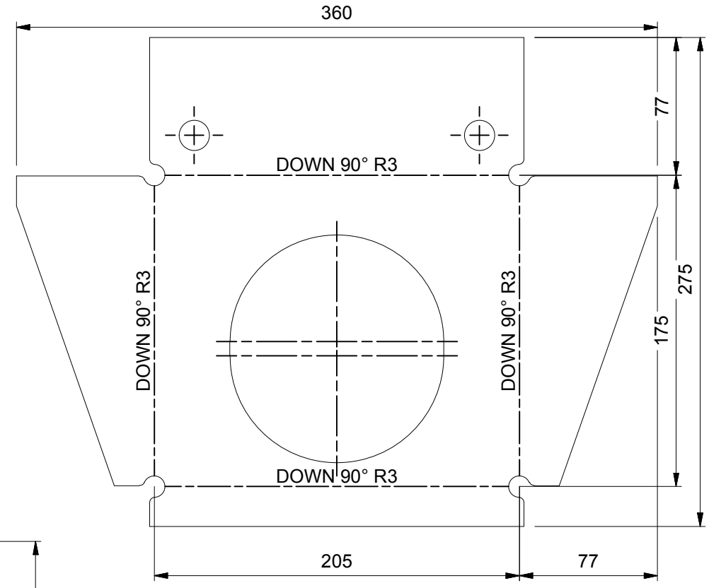
Flat pattern ( 1 : 3 )
