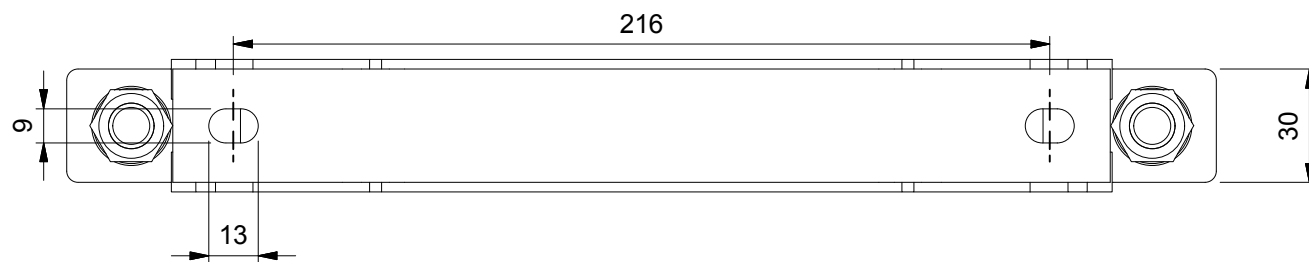
A-A ( 1 : 2 )
